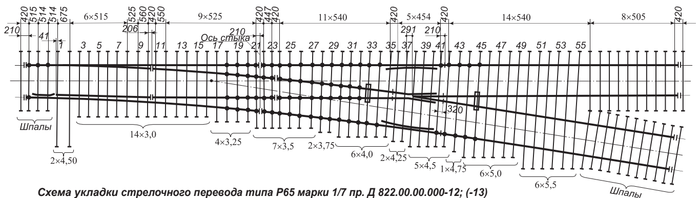
Схема укладки стрелочного перевода типа Р65 марки 1/7 пр. Д 822.00.00.000-12; (-13)
