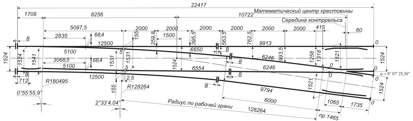
Схема геометрических размеров стрелочного перевода типа Р65 марки 1/7 пр. Д 822.00.00.000-12; (-13)
